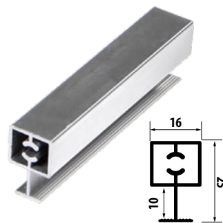
Поперечина средняя
